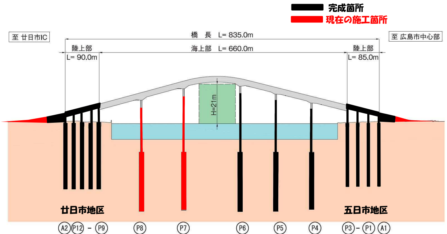
海上部の橋脚工事の状況 (4/22)
