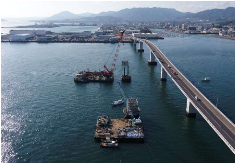
海上部の橋脚工事の状況 (1/9)
