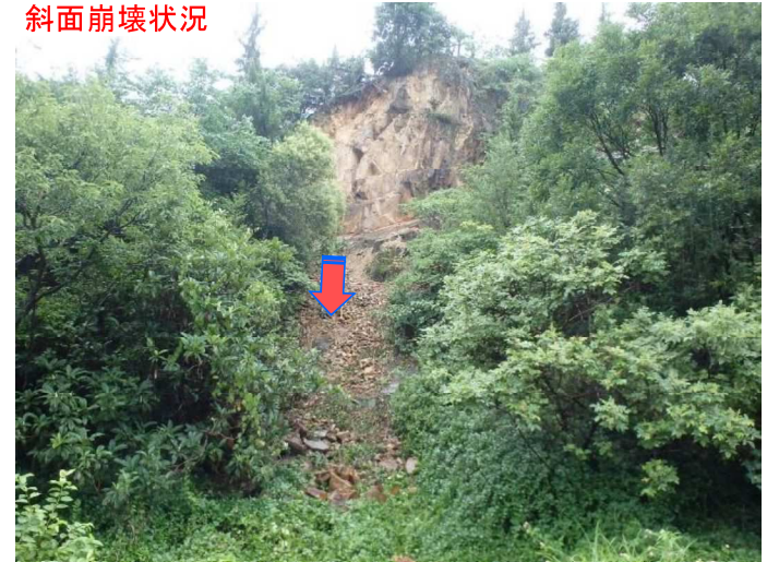
崩壊土砂流出状況
