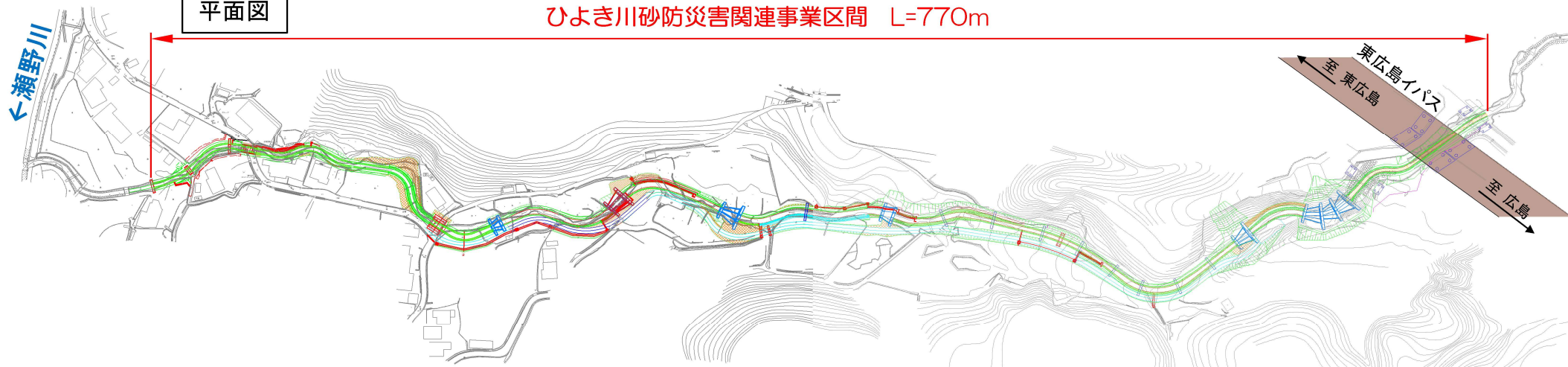
ひよき川 砂防災害関連事業 完了 (R5.3)
