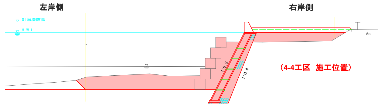
標準断面図 (A-A)
