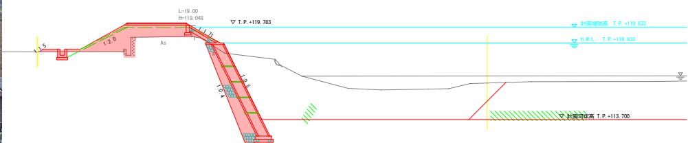
標準断面図 (A-A)
