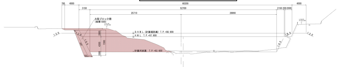
標準断面図 (A-A)
