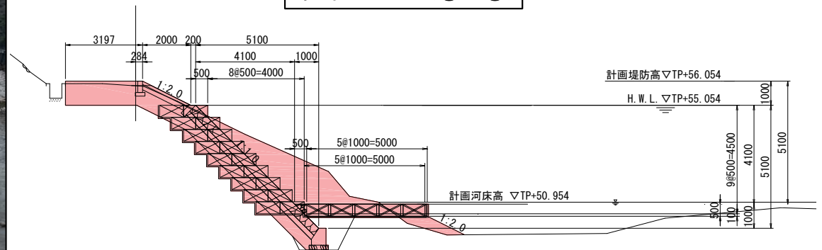
標準断面図 (A-A)
