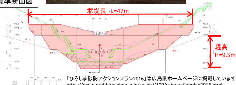
標準断面図
