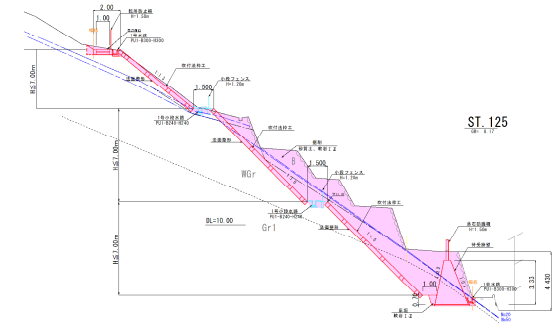
標準断面図
