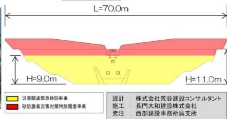
堰堤一般図
