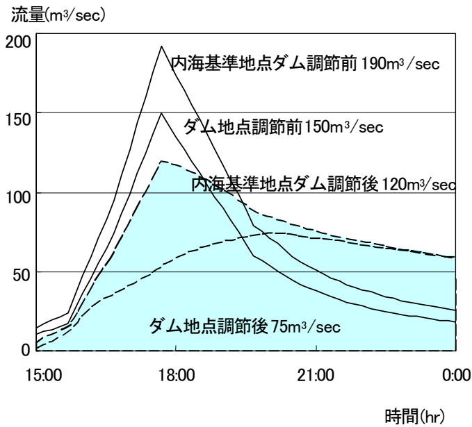
洪水調整効果図
