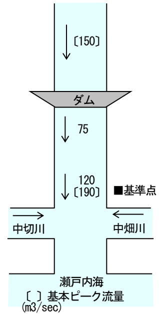
流量配分図
