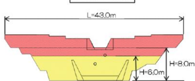
■堰堤一般図
