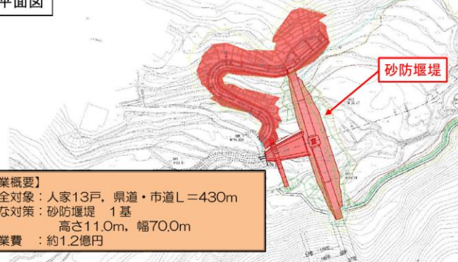
堰堤一般図
