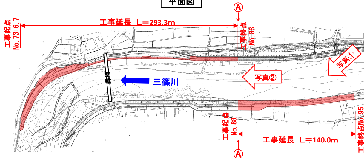
平面図
