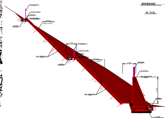
標準断面図
