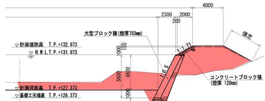
標準断面図 (A-A)
