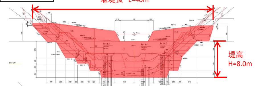
標準断面図
