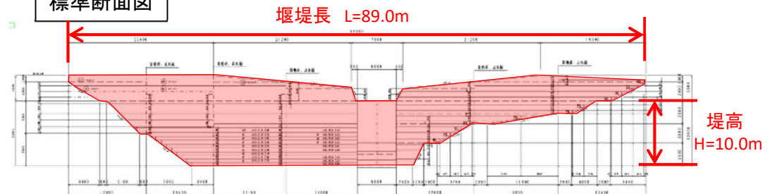
標準断面図
