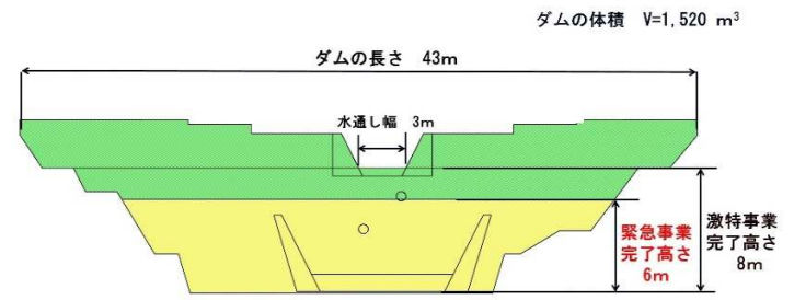
ダブルウォール工法【ソイルセメント】
