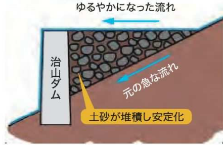
溪流を横から見た図
