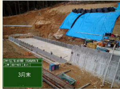
(5)2020.3 本堤工打設状況①
