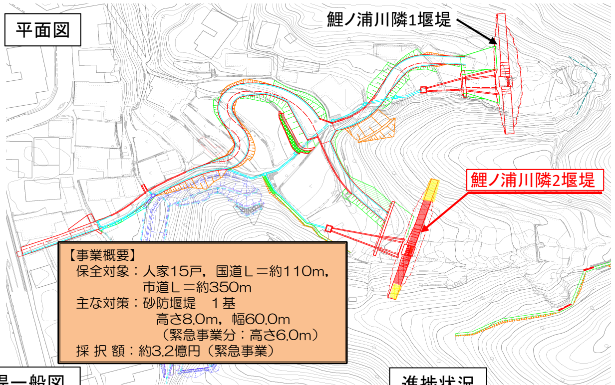
堰堤一般図
