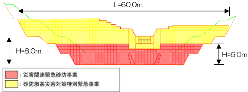
堰堤一般図
