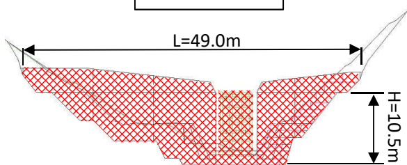
堰堤一般図
