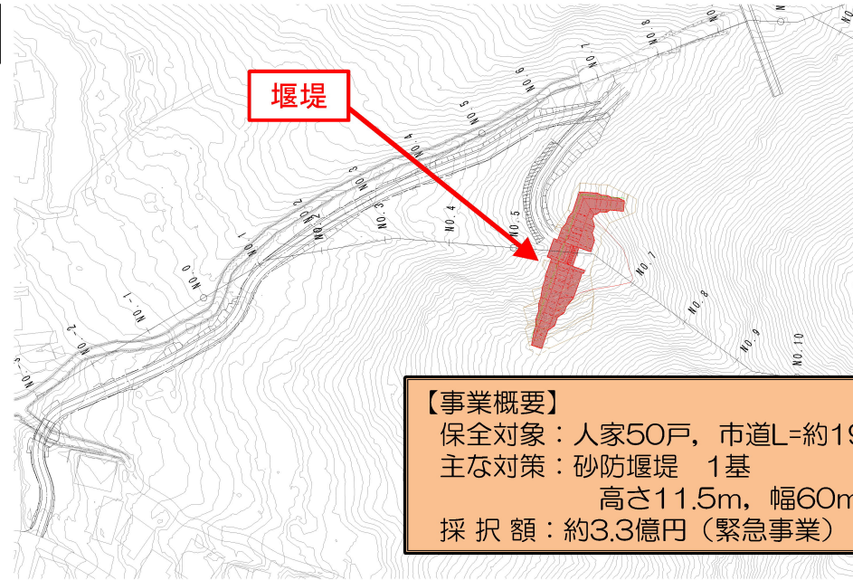
堰堤一般図
