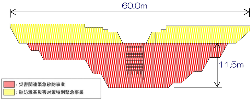
堰堤一般図
