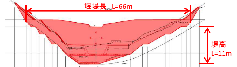
正面図
