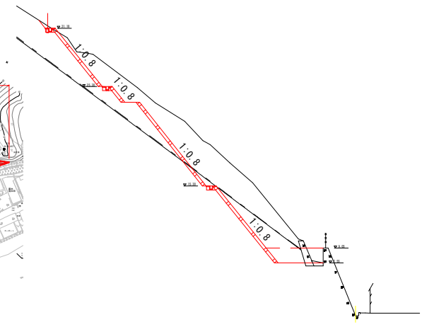
標準断面図
