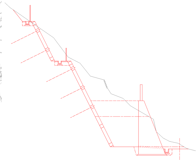
標準断面図
