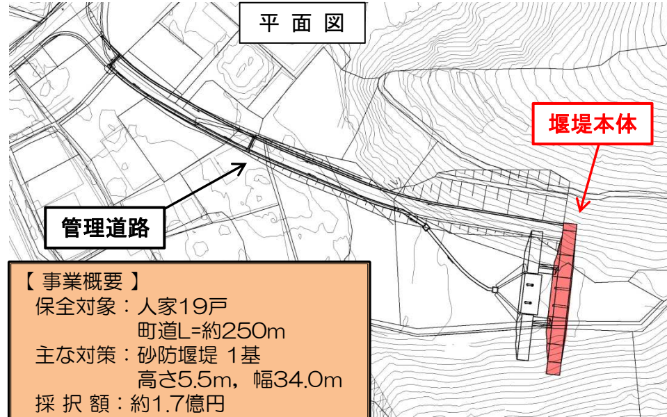
堰堤一般図
