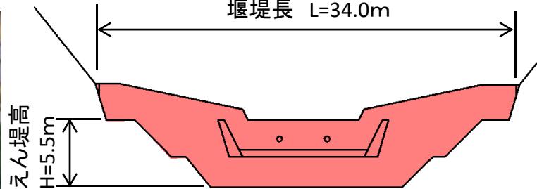
堰堤一般図
