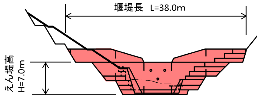
堰堤一般図
