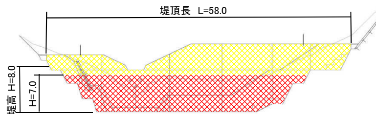
堰堤一般図
