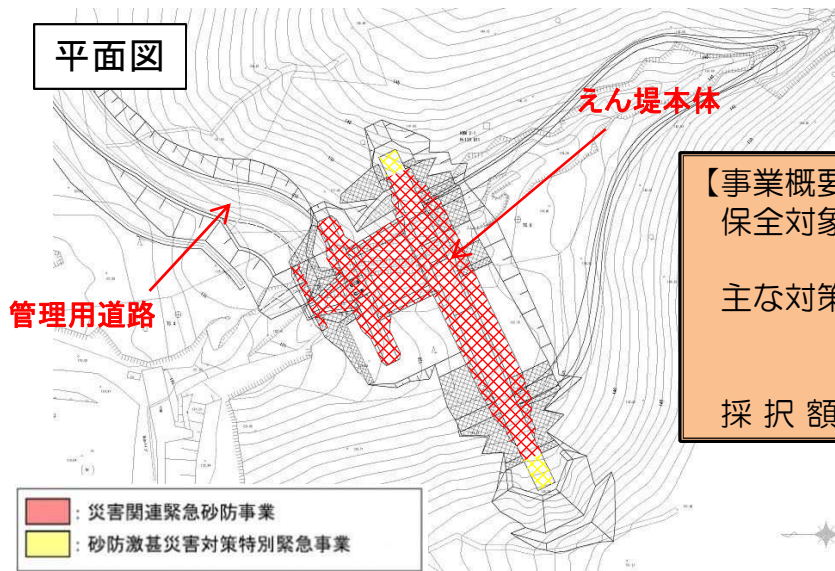
堰堤一般図
