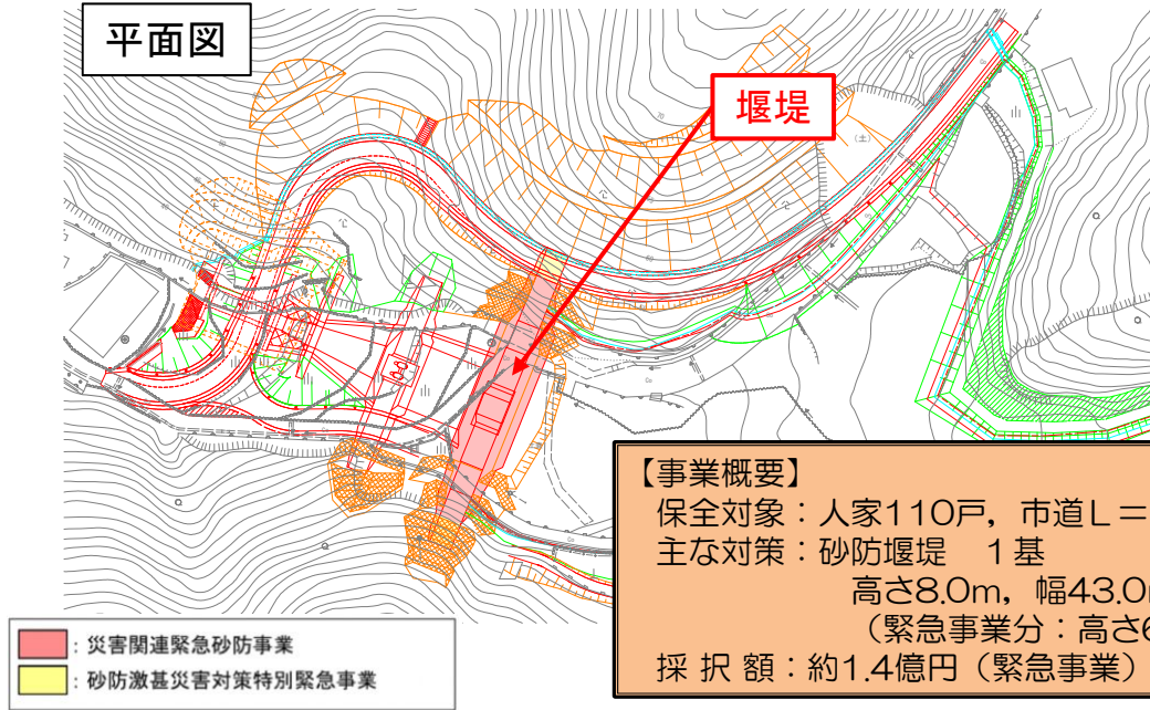
堰堤一般図
