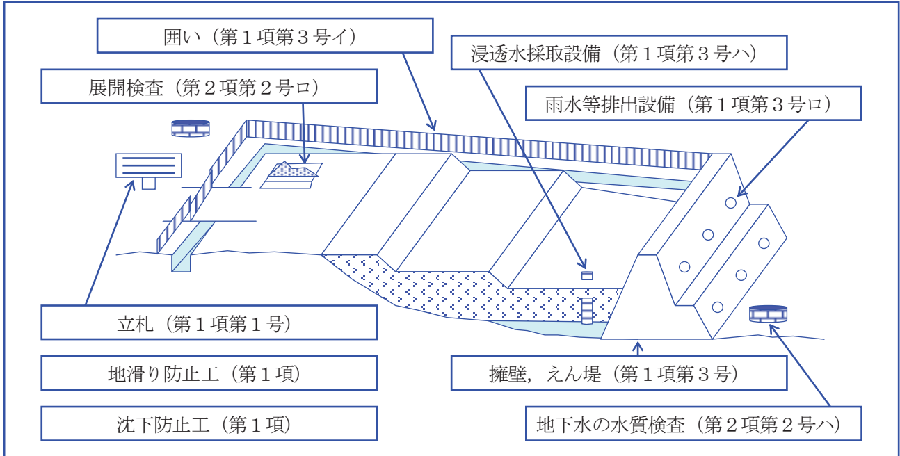
図表 26 安定型最終処分場の構造等（最終処分基準省令第2条）
