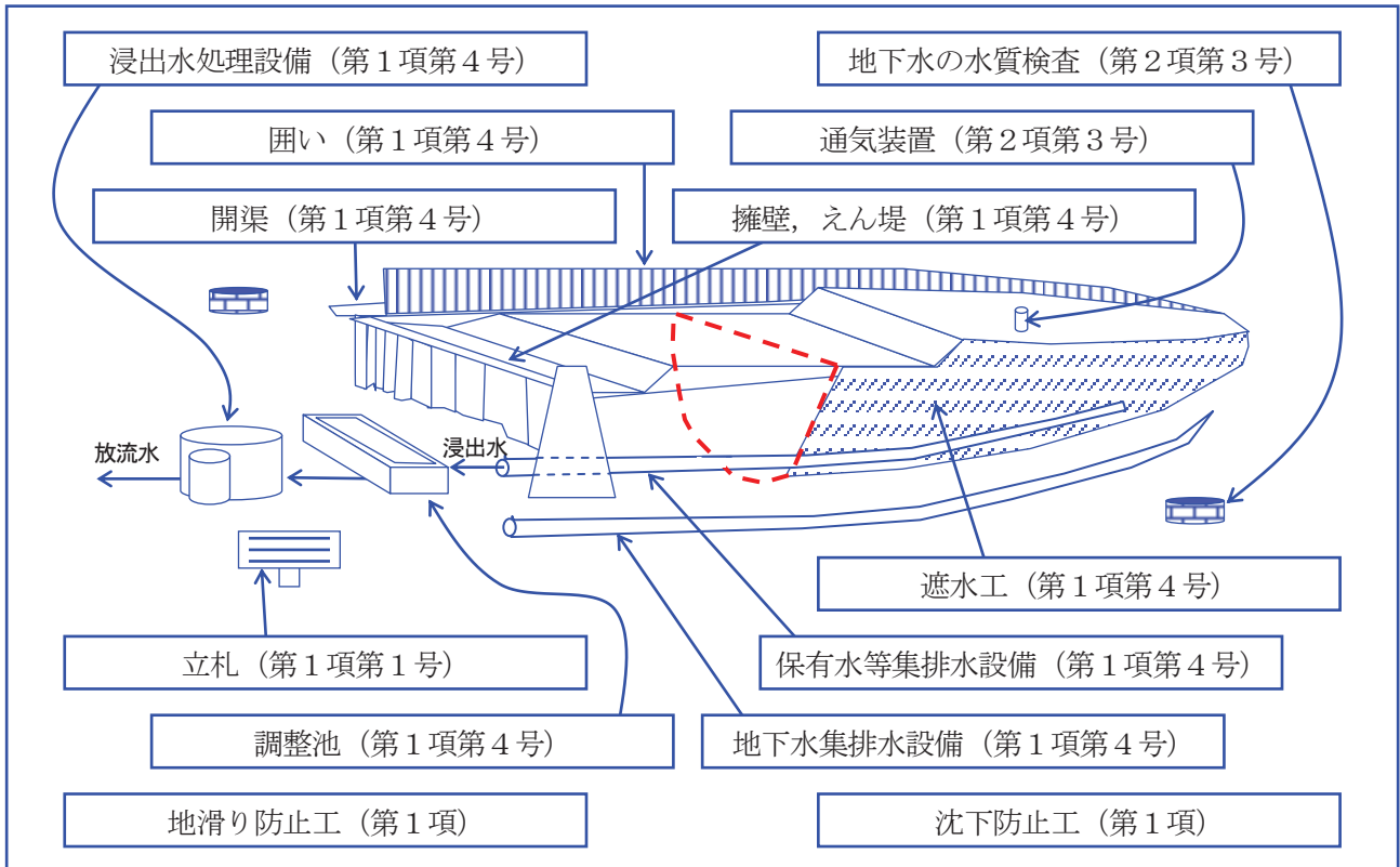
図表 27 管理型最終処分場の構造等（最終処分基準省令第2条）
