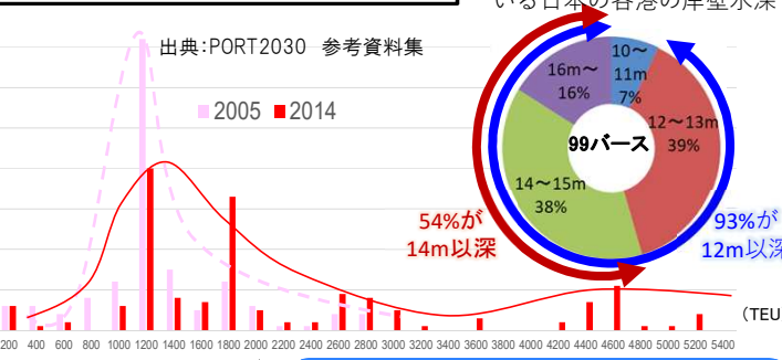
日本に寄港する東南アジア航路の船型変化
