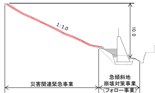
標準断面図
