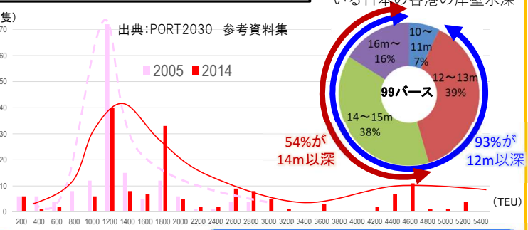
日本に寄港する東南アジア航路の船型変化
