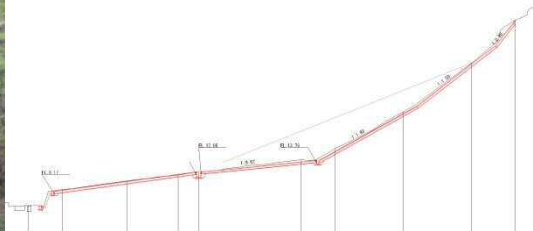
標準断面図
