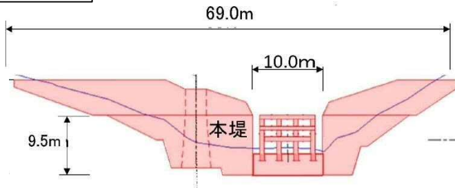
堰堤一般図
