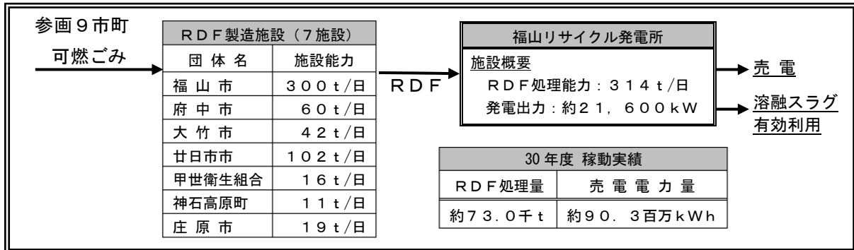
図表 2-1-7 福山リサイクル発電事業の概要
