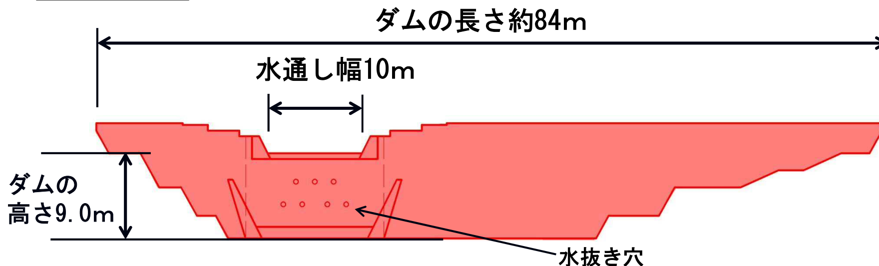
正面図
