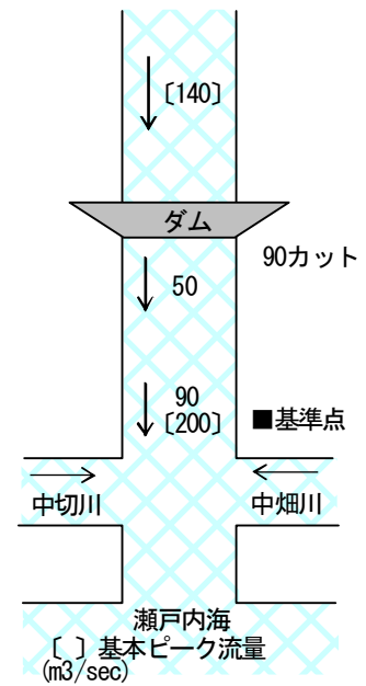
流量配分図
