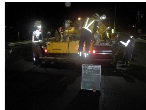
フィニッシャーによる敷均し
