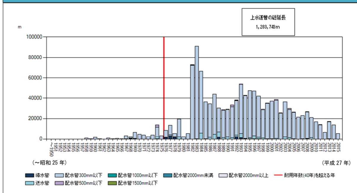
上水道（管）の竣工年別の分布状況（延長）
