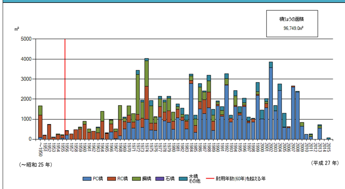
橋りょうの竣工年別の分布状況（面積）
