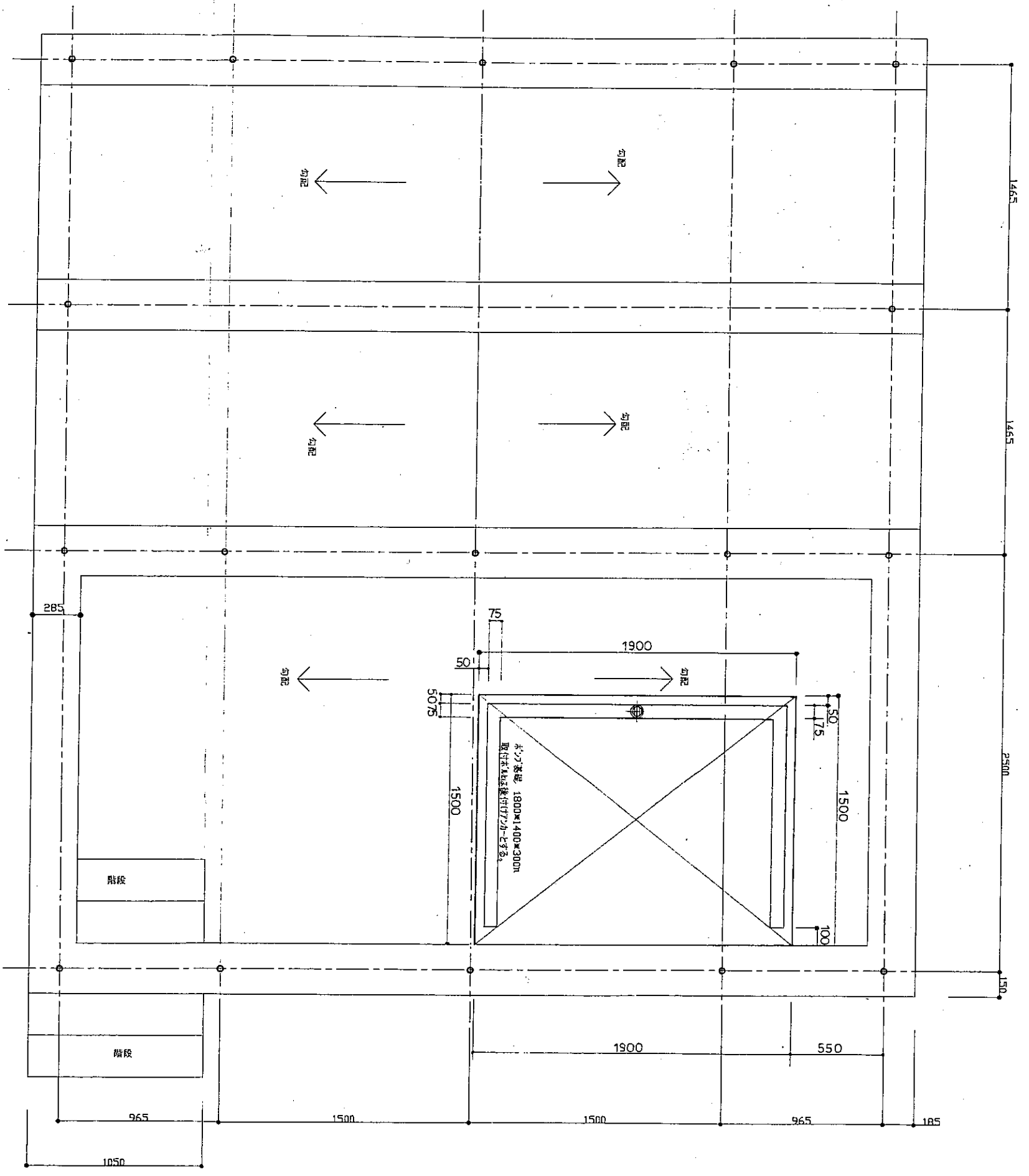
基礎平面図
