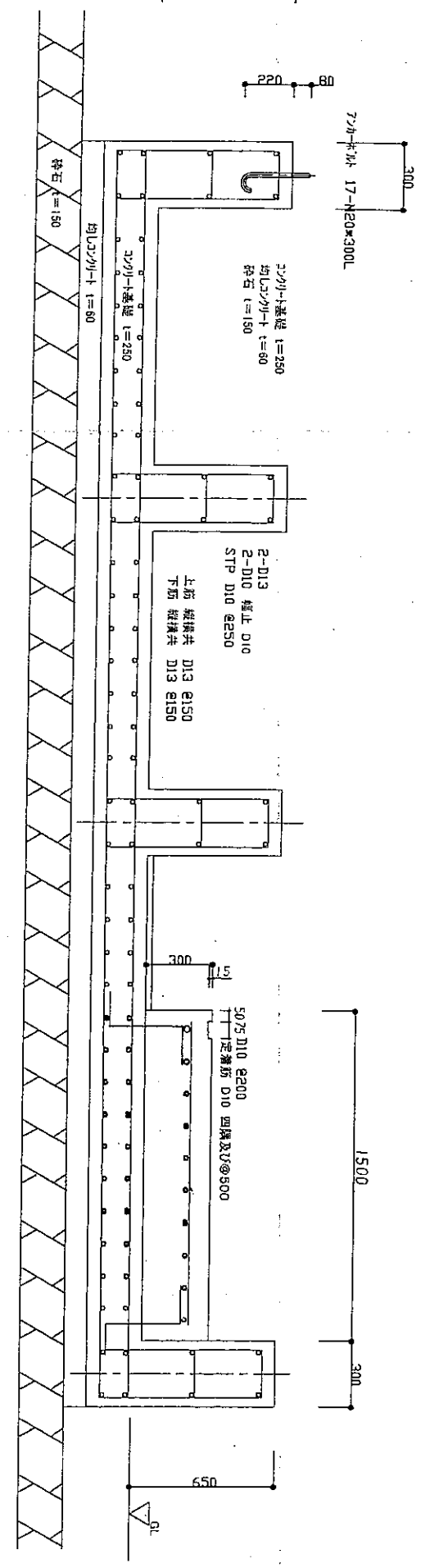
基礎断面図
