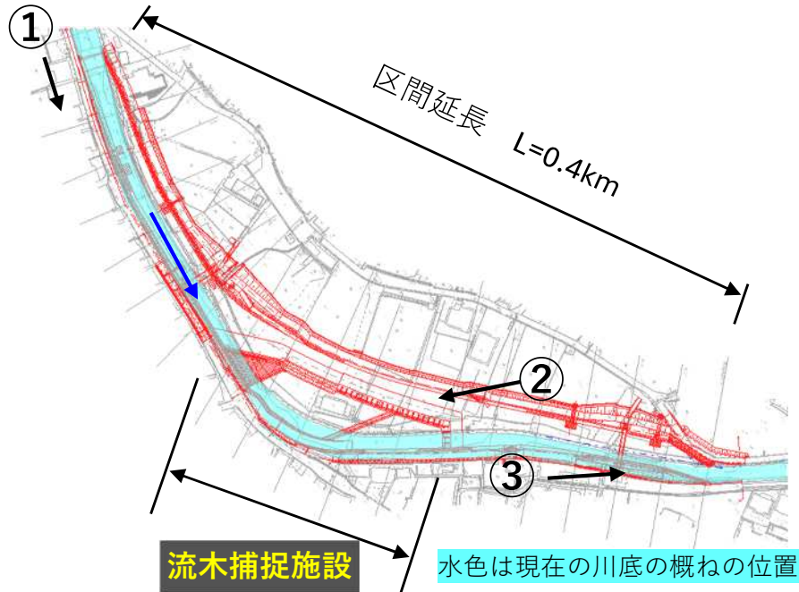
流木捕捉工区平面図
