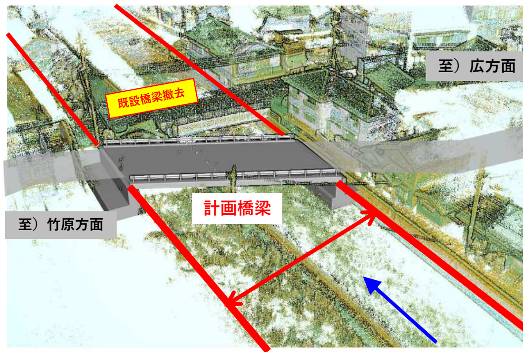
広島県 インフラマネジメント基盤 Doboxに現地での測量成果を合成
