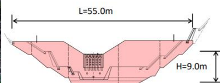
堰堤一般図
