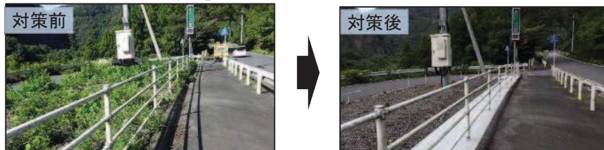
【河道浚渫・伐木 対策事例】
