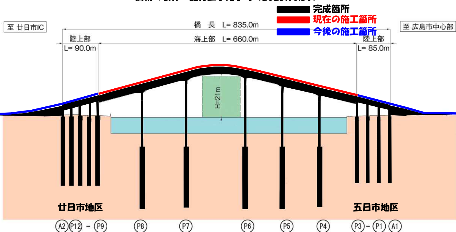
橋桁の製作・据付工事完了時（2025.10.30）
