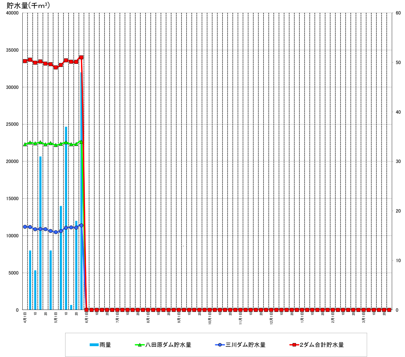
八田原ダム、三川ダムの貯水状況グラフ(令和7年度)
