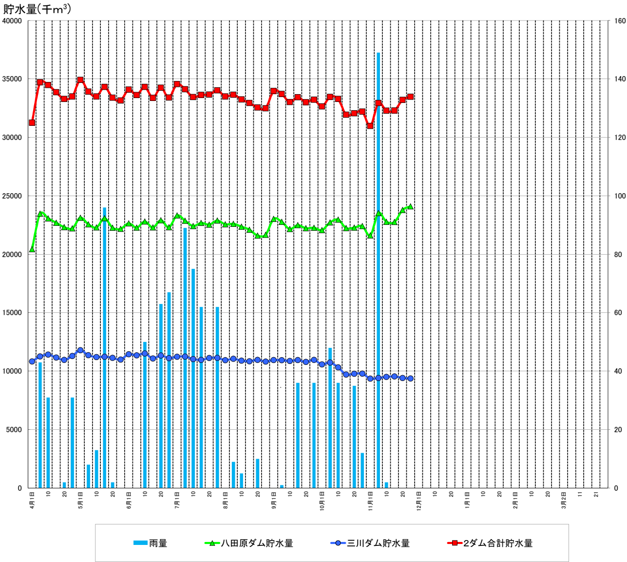
八田原ダム、三川ダムの貯水状況グラフ(令和6年度)
