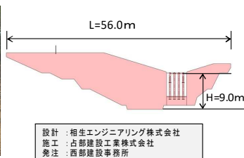
堰堤一般図
