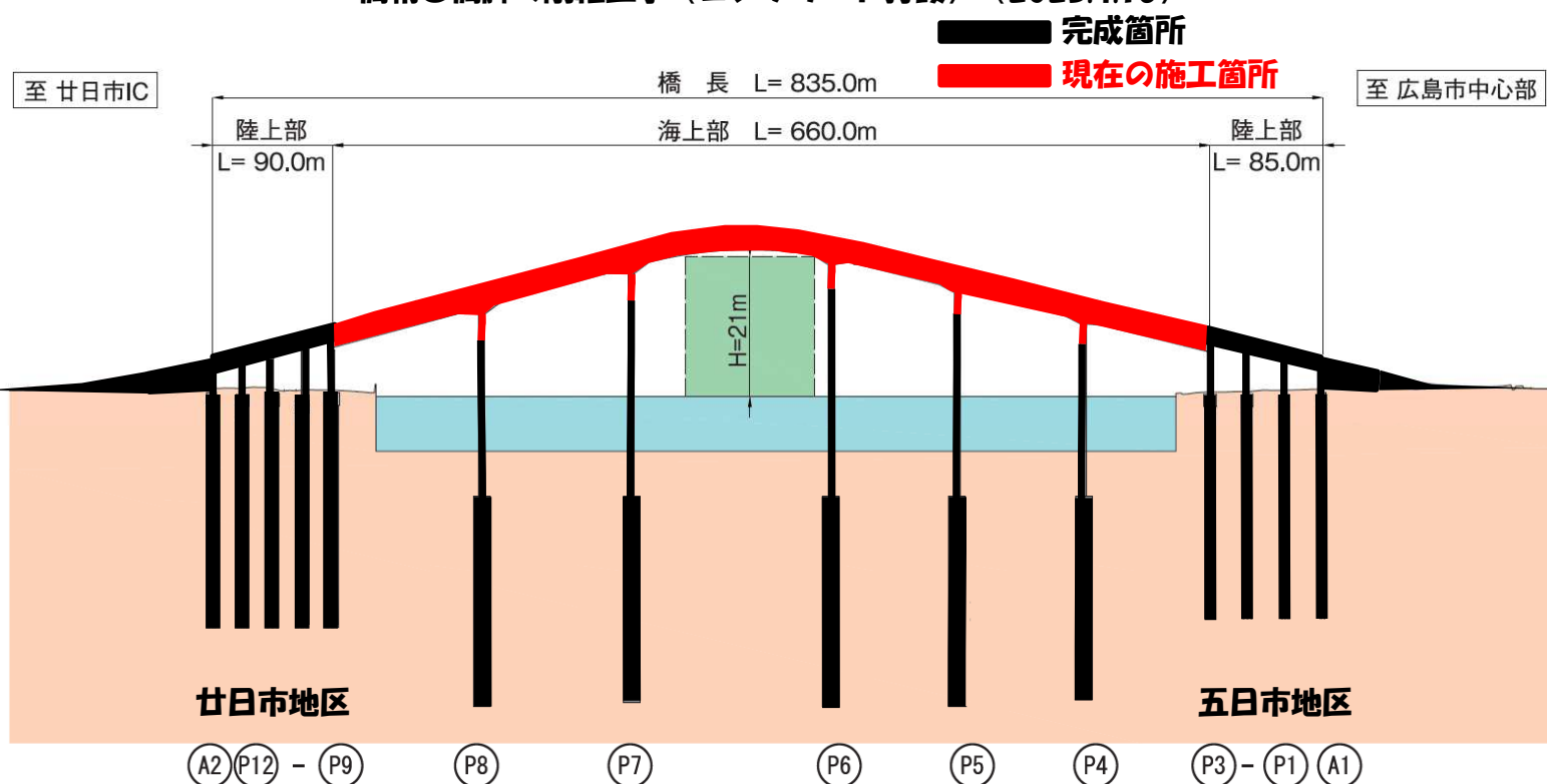
橋桁と橋脚の剛結工事（コンクリート打設）（2025.4.16）
